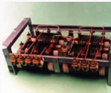
Блоки резисторов БФК ИРАК
