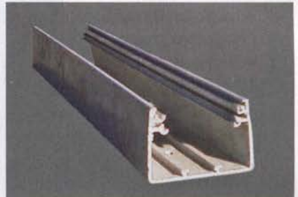
Фото 2. Основа стойки — отрезок кабель-канала сечением 40 × 75 мм и длиной 800 мм.
