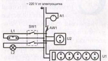
Рис. 2. Принципиальная схема соединений: AW1 — автоматический выключатель 15 А; SW1 — двоярный выключатель; L1 — люминесцентный светильник общего освещения мастерской; L2 — лампа местного освещения над электроточилом; U1 — электроудлинитель на пять розеток; U2 — розетка.
