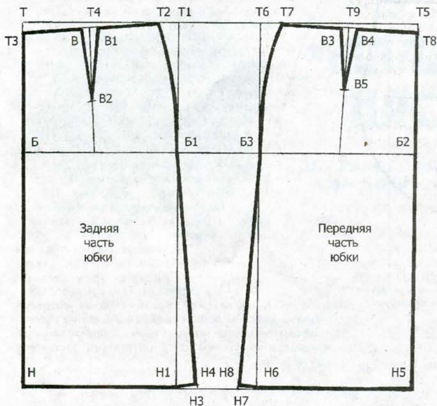
Чертеж основы (заднее и переднее полотнище юбки)
