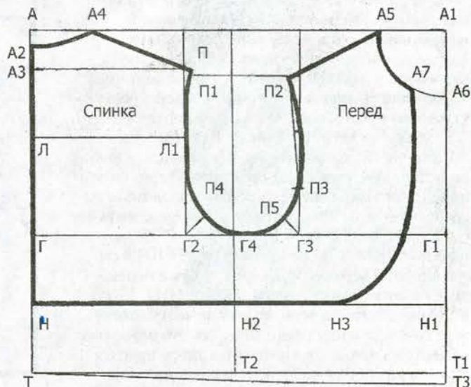
Чертеж жилета (перед, спинка)
