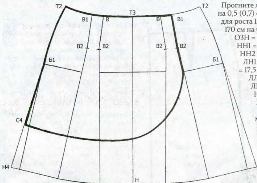
37_1_Чертеж верхней части юбки (заднее полотнище)
