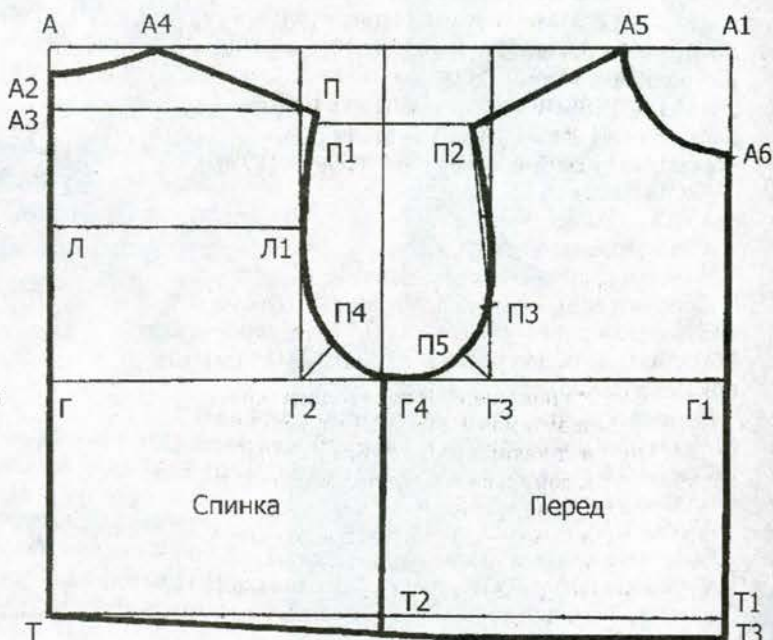
Чертеж основы (спинка, перед)
