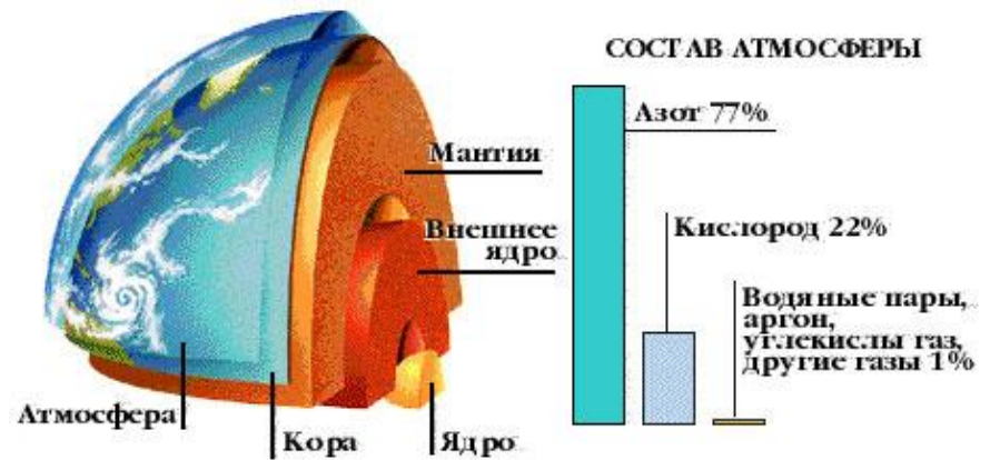
Схематическое изображение внутренней структуры земного шара
