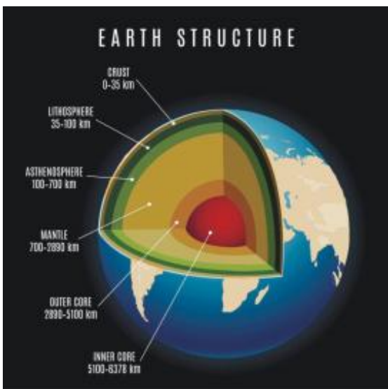
Схематическое изображение внутренней структуры земного шара
