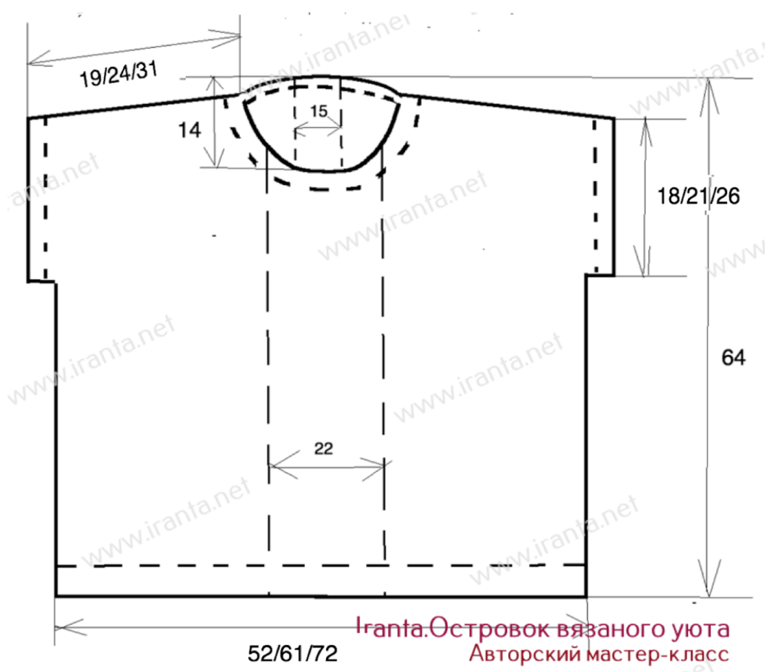
СХЕМА ДЖЕМПЕРА с удлиненной полукруглой спинкой
