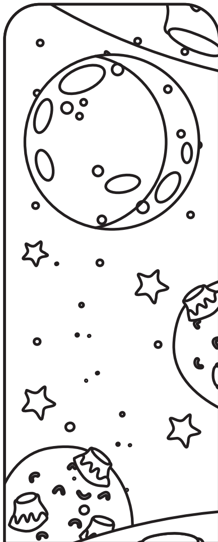
WANING GIBBOS
